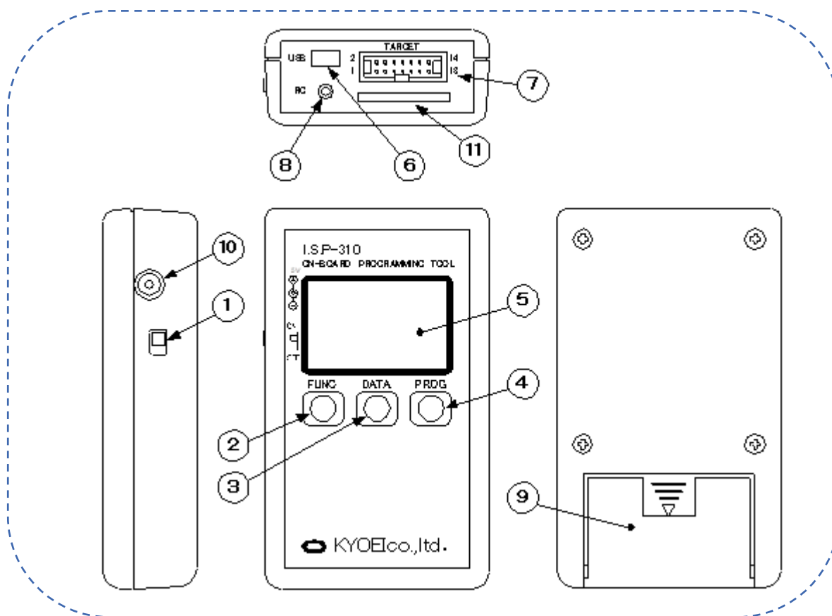
Fig 1 各部の外観と主な機能
