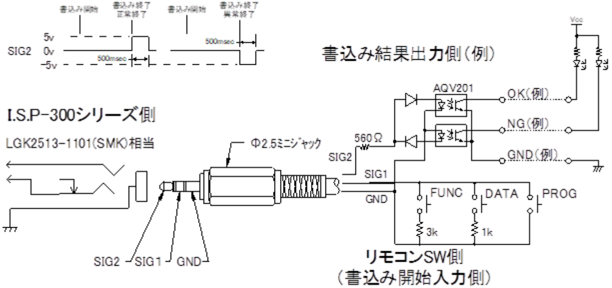
Fig 6 スイッチ操作リモート接続
